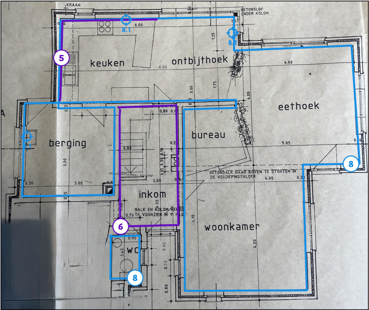
Legende van plan 1.2: Gelijkvloers - Muren
