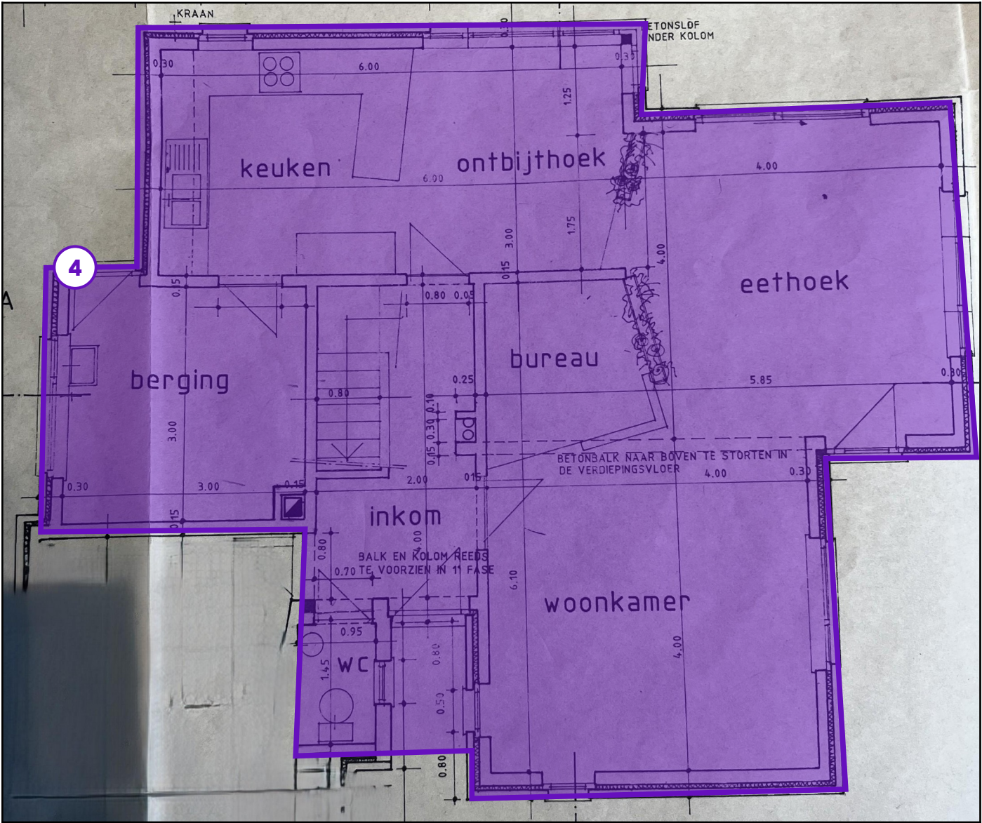
Legende van plan 1.1: Gelijkvloers - Vloeren
